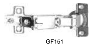
GF151
